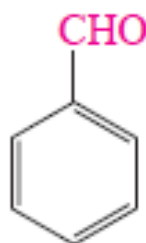
benzenkarbaldehid (benzaldehyd)
