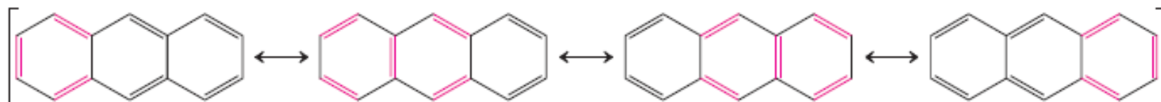
Rezonancija fenantrena
