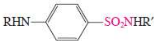
opšta struktura
