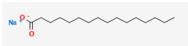
natrijum-palmitat
