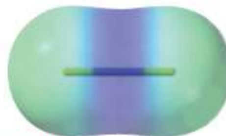
nitronijum-jon
