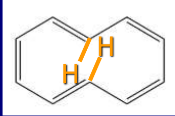
trans,trans izomer
