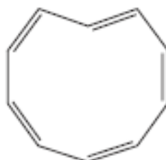
trans,cis,cis,cis,cis - -[10] anulen
