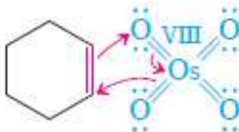
adicija osmijum-tetroksida
