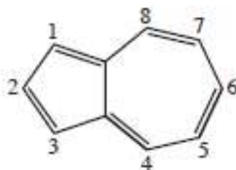
azulen
