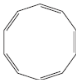
cis,cis,cis,cis,cis - -[10] anulen
