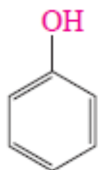
benzenol (fenol)
