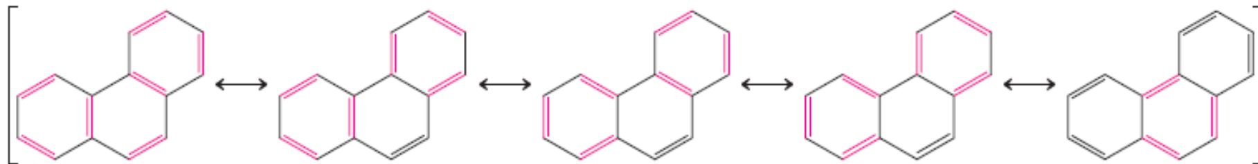
Rezonancija fenantrena
