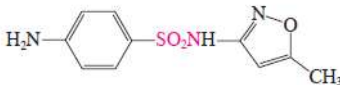
sulfametoksazol (gantanol)
