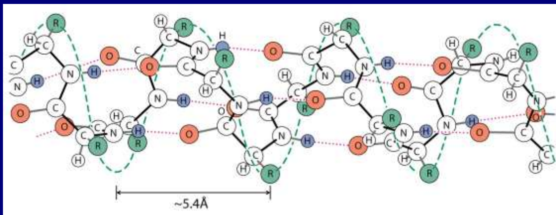
Polipeptid
