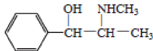
pseudoefedrin
