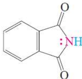
1,2-benzendikarboksimid (ftalimid)
