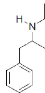
apetenil
