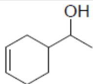
1-(cikloheks-3-enil)etanol
