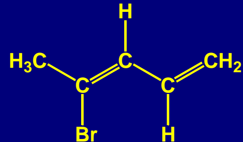
( Z )-4-brom-1,3-Pentadien
