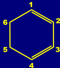
1,3-cikloheksadien
