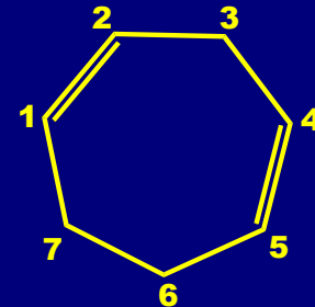
1,4-cikloheptadien
