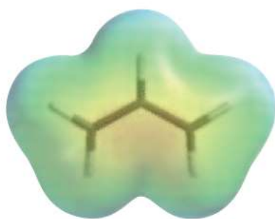
radikal
