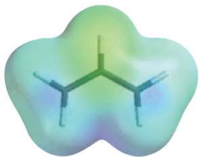
katjon
