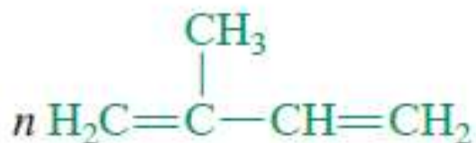
2-metil-1,3-butadien
