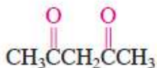
2,4-pentan dion (acetilaceton) ( \beta -diketon)
