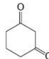
1,3-cikloheksandion
