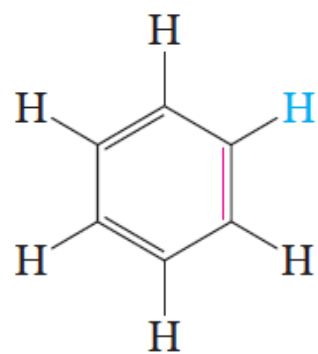
benzen
