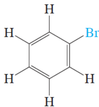
brombenzen
